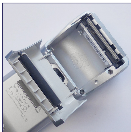
2. Druckerklappe öffnen
